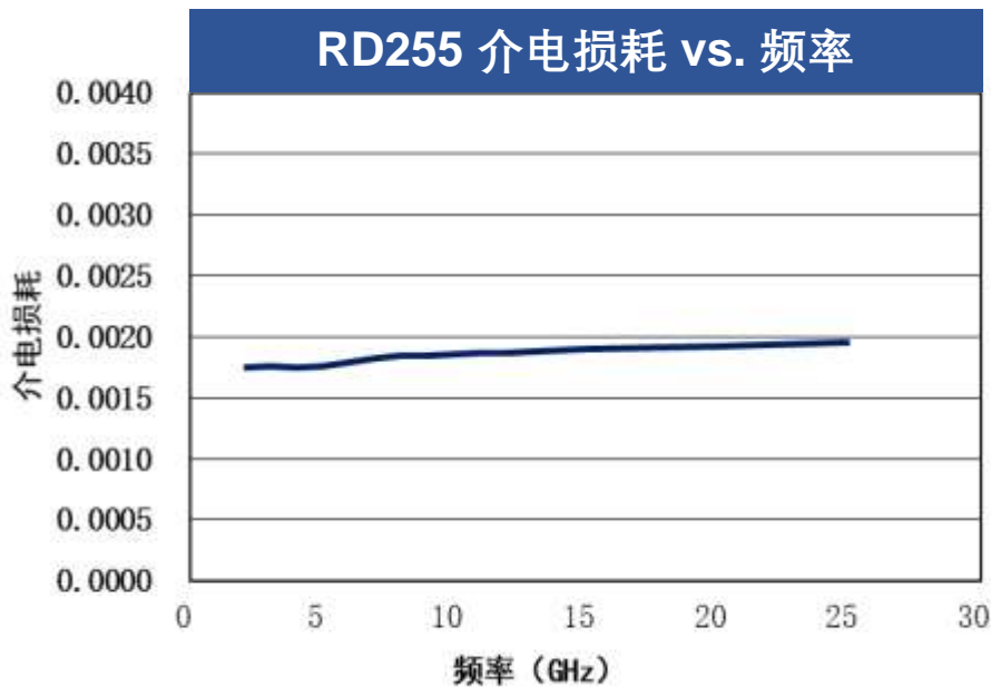
图 2 证明了介电损耗随频率变化的稳定性 这个特性证明了睿龙 RD255 材料跨频率的固有稳定性，为高频应用中信号完整性作为整体性能关键性部分提供了一个稳定的平台。
