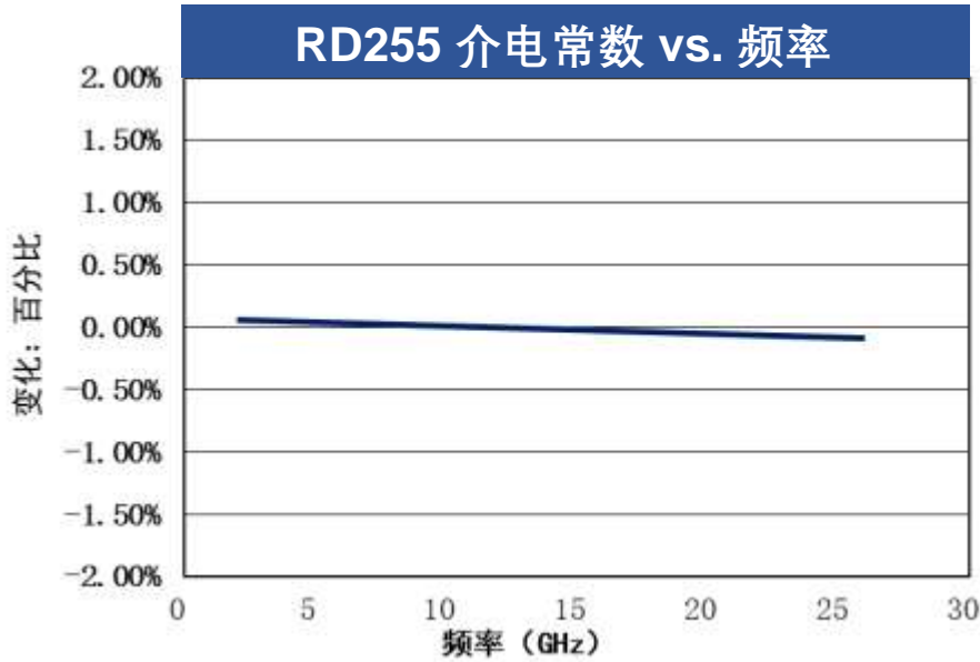
图 1 证明了介电常数随频率变化的稳定性 这个特性证明了睿龙 RD255 材料跨频率的固有稳定性，从而简化整个电磁频谱范围的最终设计，RD255 介电常数在整个频率范围的稳定性确保设计及放大的稳定性。
